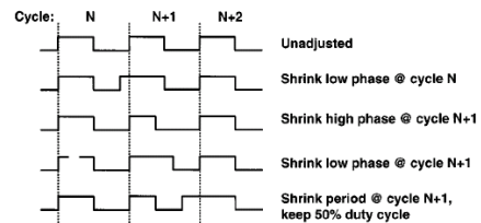
Fig. 16. ODCS capabilities.
